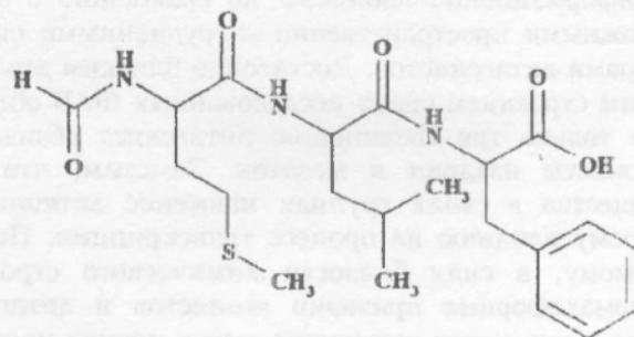
MLP
