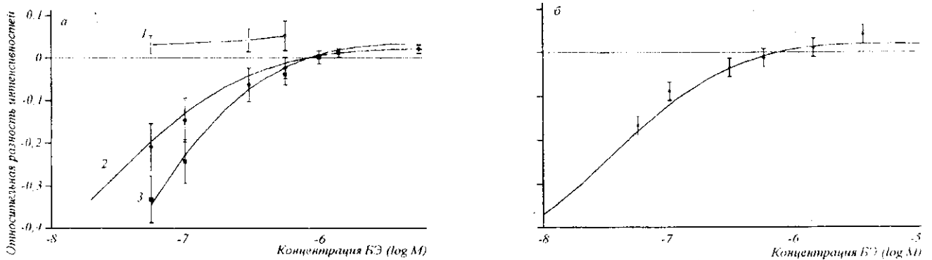
Рис. 2. А — зависимость относительного изменения флюоресценции политенных хромосом от концентрации красителя (1 — при действии ДНКазы I, добавленной после топоизомеразы I; 2 — при действии топоизомеразы I; 3 — при действии ДНКазы I на хромосомы IV без ядрышек); Б — относительное изменение флюоресценции политенных ядер при действии ДНКазы I после обработки панкреатической РНКазой
